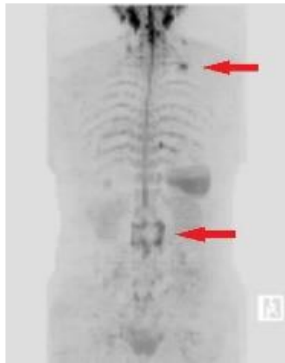
DWIBS画像
